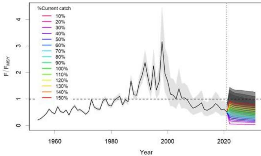
圖 50. 基礎情境(S0)下歷年及未來投射之西北太平洋鬼頭刀漁獲死亡率相對於 MSY 水準下漁獲死亡率(F/F MSY )之變動趨勢。
