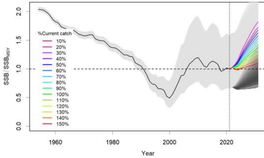
圖 49. 基礎情境(S0)下歷年及未來投射之西北太平洋鬼頭刀親魚量相對於 MSY 親魚量水準(SSB/SSB MSY )之變動趨勢。
