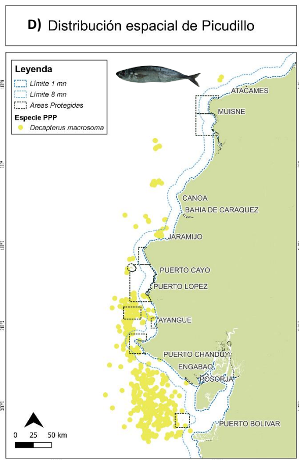
Figura c1. Distribución espacial de las especies a) botella, b) chuhueco, c) macarela y d) picudillo
